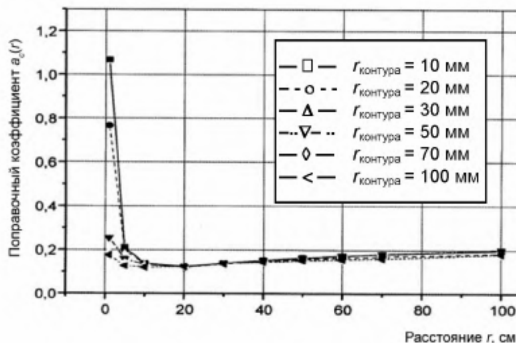
Рисунок С.5 – Поправочный коэффициент a_c(r_1) для полей с удельной электропроводностью 0,1 \text{ См/м} и датчиком площадью A_{\text{датчик}} = 100 \text{ см}^2 для модели тела человека (применяются шкалы значений пределов согласно ICNIRP [11])
