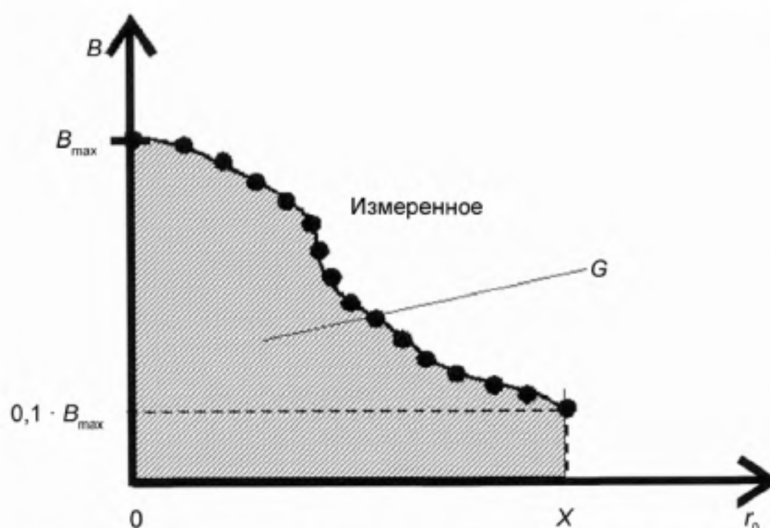
Рисунок С.2 – Градиент плотности магнитной индукции
