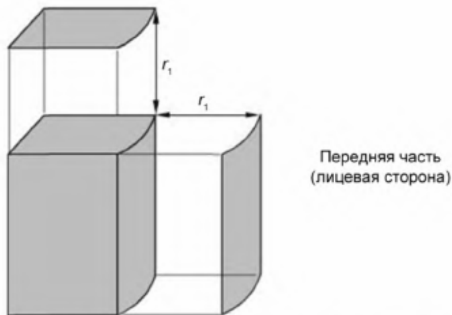
Рисунок А.1 – Измерительное положение верх/передняя часть (см. 3.2.7)
