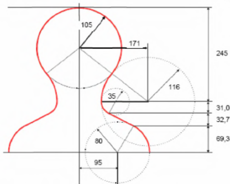
Рисунок D.4 – Детализированный чертеж модели головы и плеч
