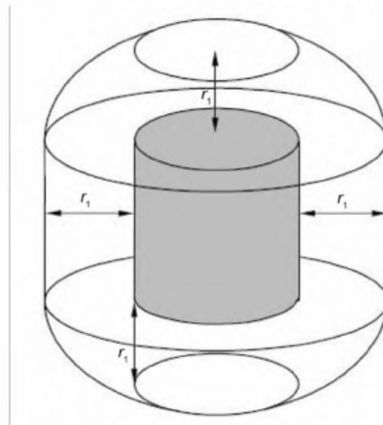
Рисунок А.2 – Измерительное положение вокруг (см. 3.2.7)
