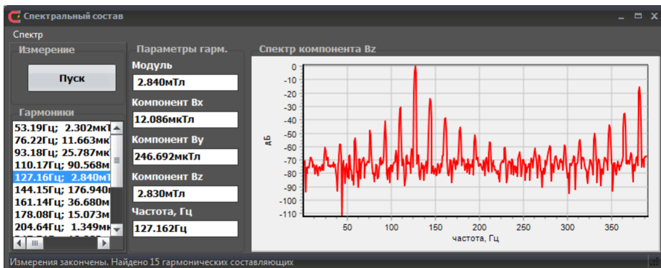
Рисунок П.10. Окно «Спектральный состав»
