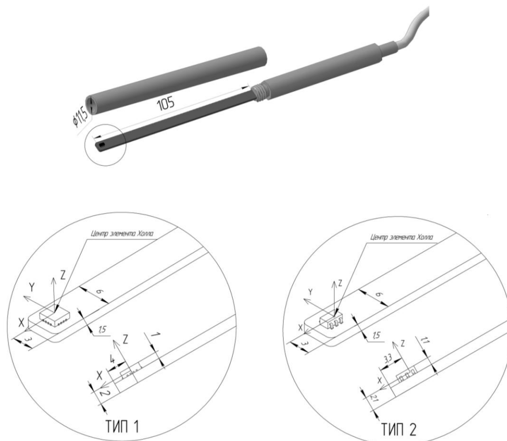
Рисунок 1.1. Вид измерительного зонда (тип 1, тип 2), направления осей X, Y, Z
