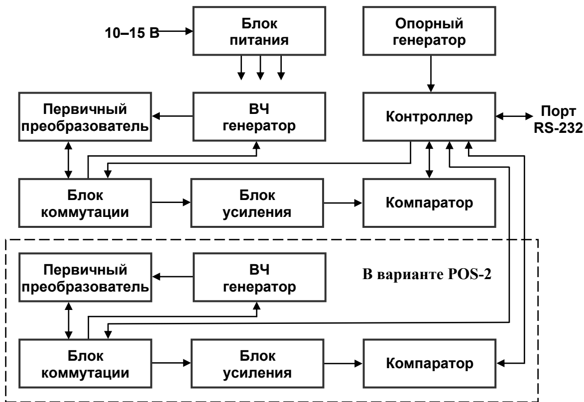
Рис. 1. Функциональная схема POS-1,2
